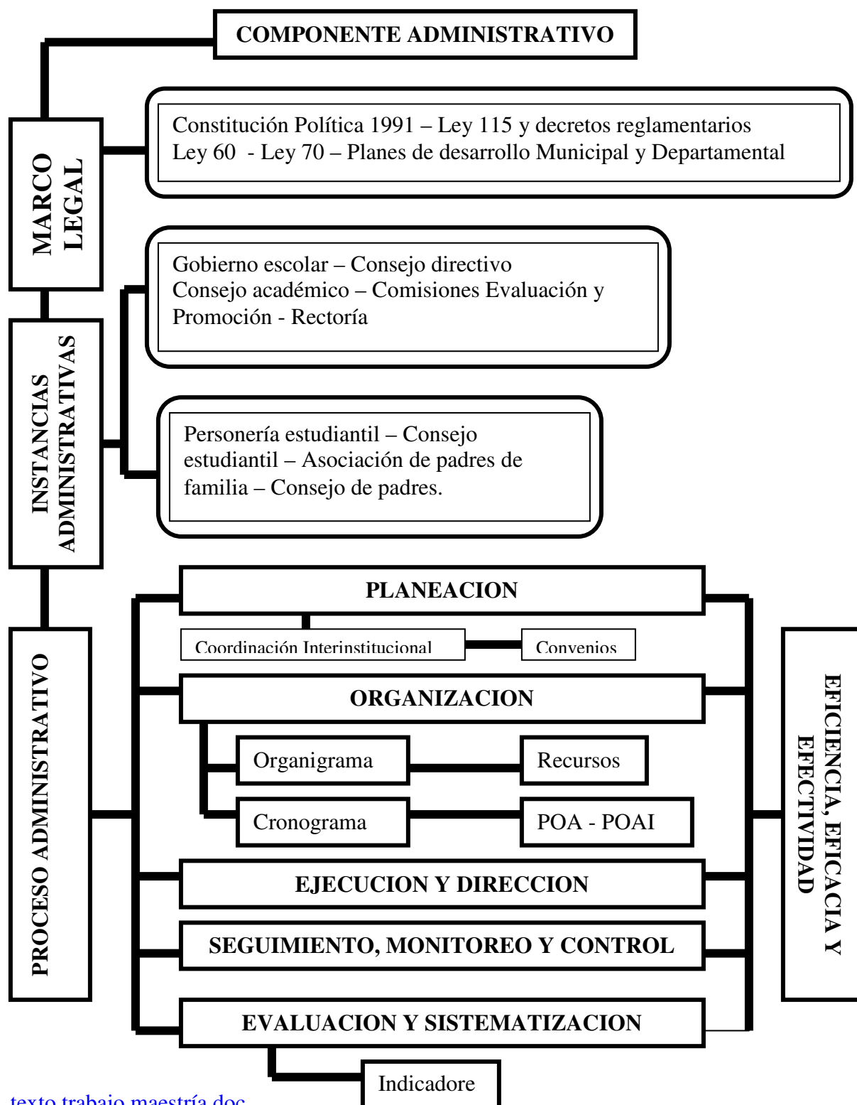
Figura 26. Componente administrativo
