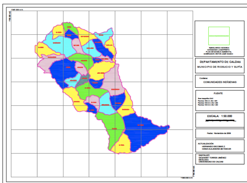
Mapa 2. Distribución comunidades Reguardo Cañamomo Lomapieta
