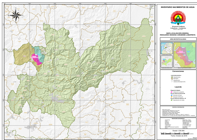
Mapa 1. Localización del Resguardo Cañamomo Lomaprieta.
