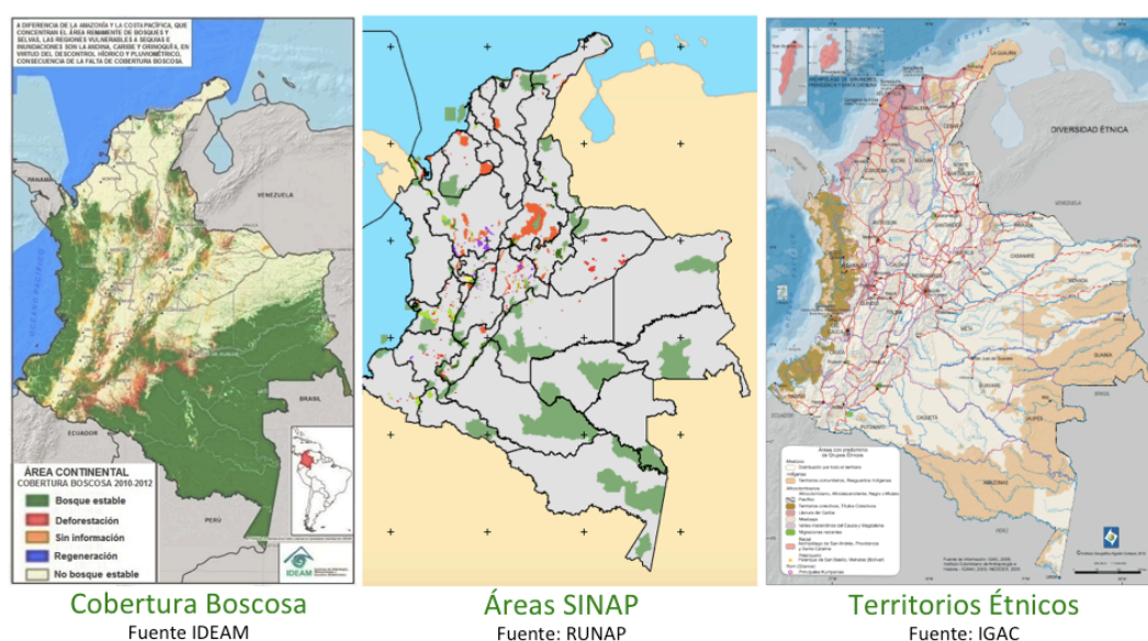
Mapa 3. Mapas de Cobertura Boscosa, Áreas SINAP y Territorios Étnicos, evidencia del cruce de territorios étnicos con áreas No Runap
