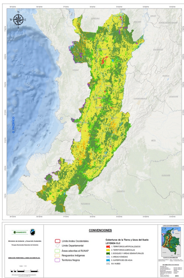
Mapa 4. Coberturas de la Tierra, Areas Runap, Territorios Colectivos de comunidades Negras y resguardos Indígenas al interior del SAO
